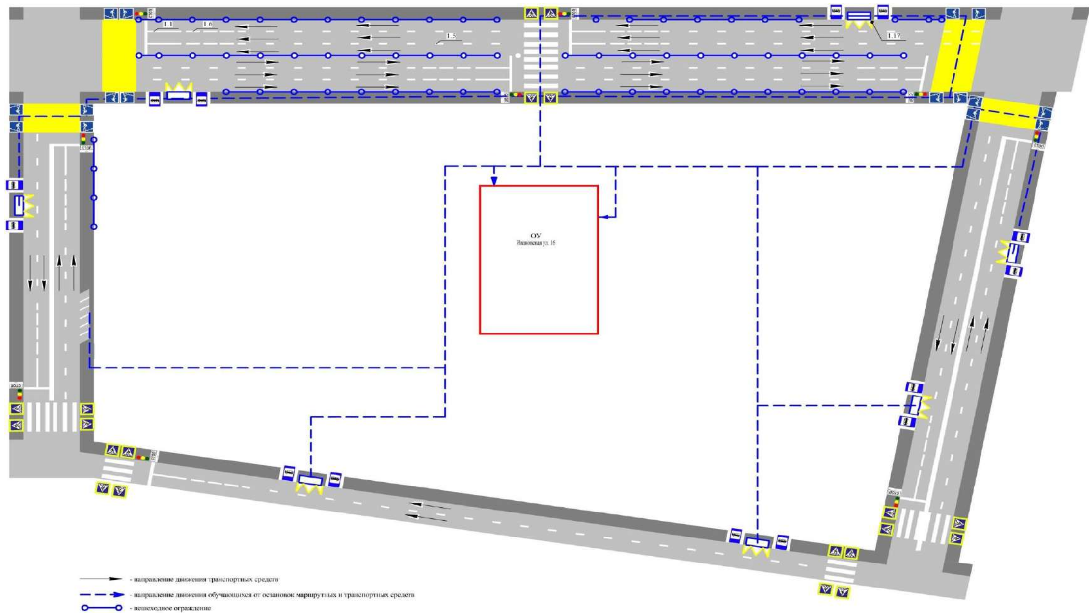
Схема организации дорожного движения в непосредственной близости от ГБПОУ Некрасовский педколледж № 1 с размещением соответствующих технических средств, маршруты движения обучающихся и расположение парковочных мест
